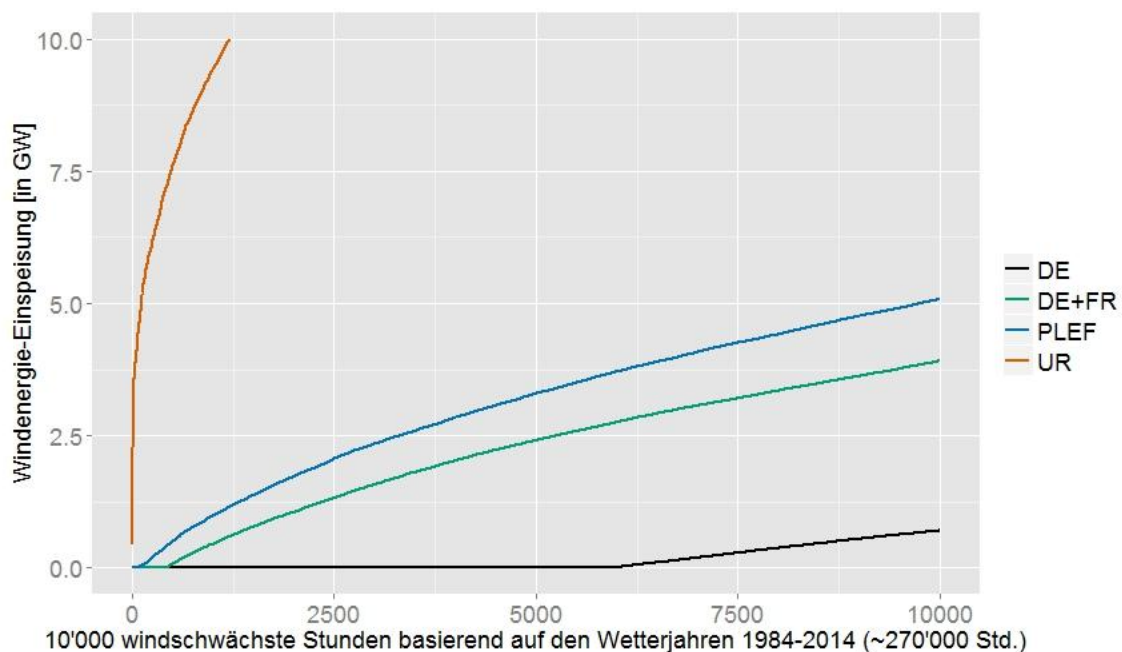
Abbildung 15: Verfügbarkeit der Windenergie in den 10'000 windschwächsten Stunden
