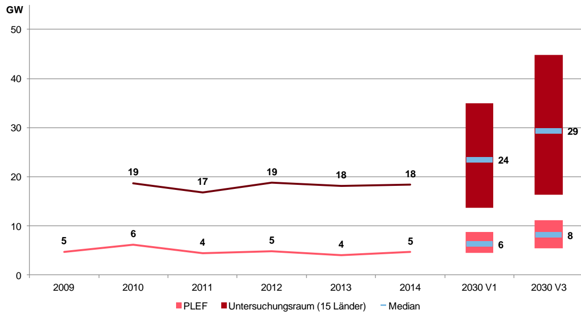
Abbildung 30: Reduktion der Residuallast in den höchsten 100 Stunden durch gemeinsame Bilanzierung im PLEF und UR 2009(10)-2014 und 2030
