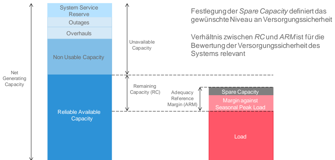
Abbildung 3: ENTSO-E Methodik Leistungsbilanzierung
