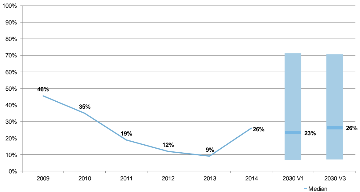
Abbildung 13: Windenergieverfügbarkeit (in Prozent der installierten Leistung) zur Stunde der Verbundhöchstlast im PLEF 2009-2014 und 2030
