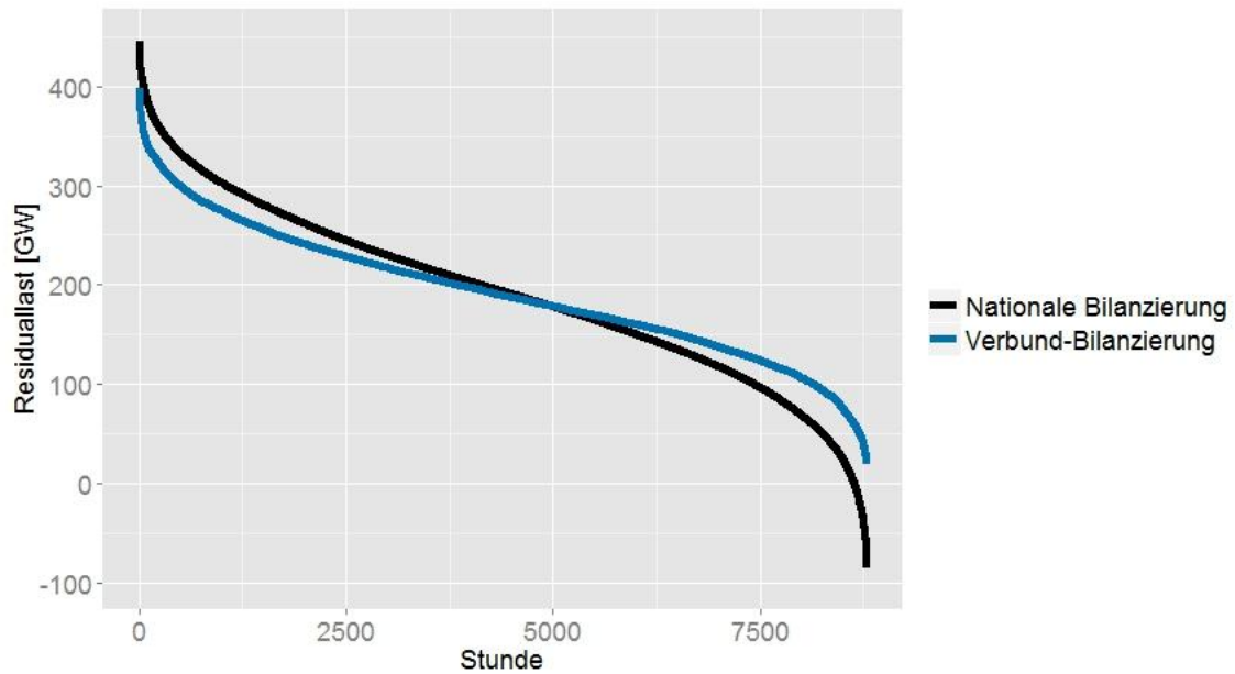
Abbildung 22: Residuale Lastdauerlinien für den Untersuchungsraum bei nationaler Bilanzierung und bei Verbund-Bilanzierung im Jahr 2030
