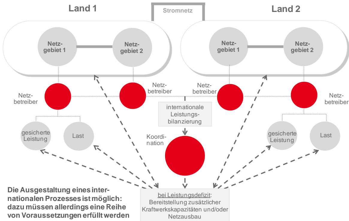
Abbildung 25: Schematische Darstellung des internationalen Leistungsabsicherungsprozesses
