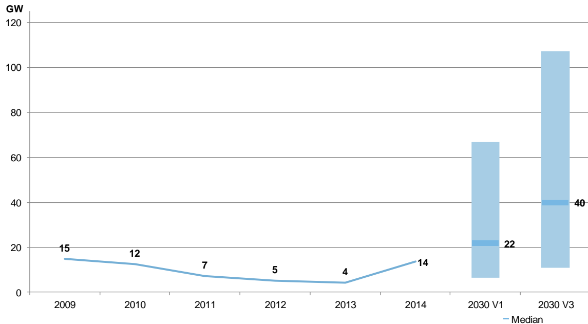
Abbildung 14: Windenergieverfügbarkeit zur Stunde der Verbundhöchstlast im PLEF 2010-2014 und 2030
