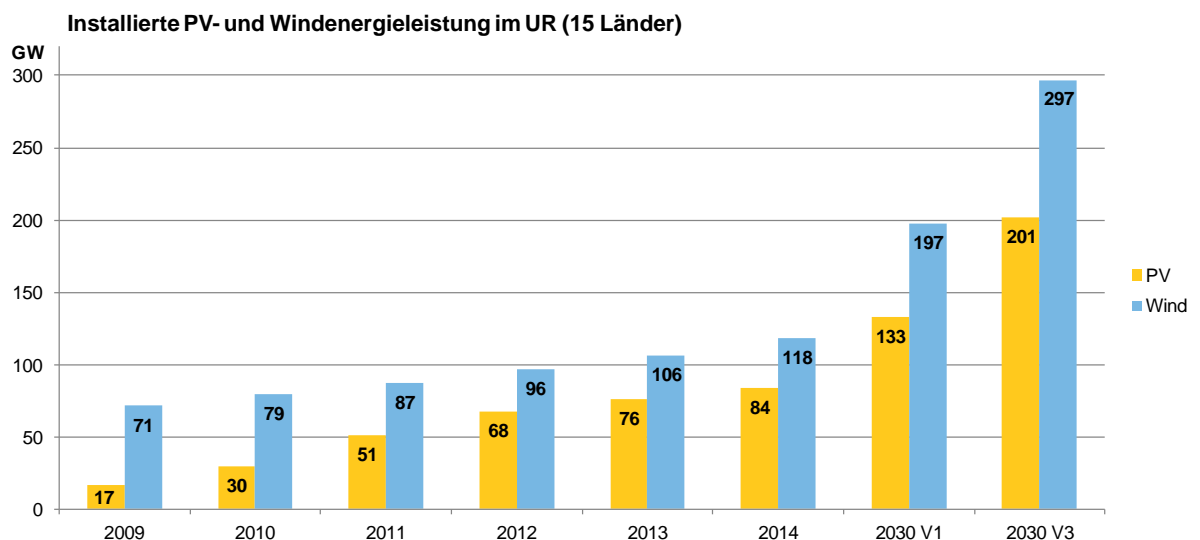
Abbildung 7: Installierte Windenergie- und PV-Leistung ex-post 2009-2014 und gemäß Szenario V1 und V3 in 2030 im Untersuchungsraum
