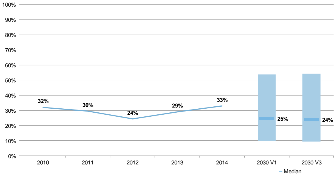
Abbildung 29: Windenergieverfügbarkeit zur Stunde der Verbundhöchstlast im Untersuchungsraum 2010-2014 und 2030
