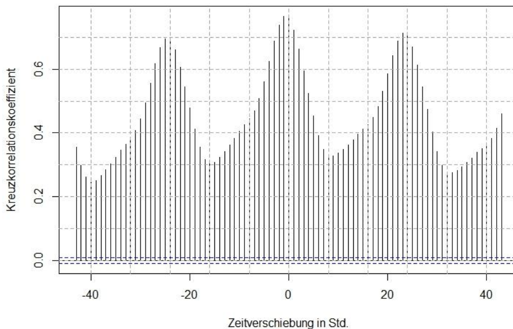
Abbildung 12: Gleichzeitigkeit der Last 2011-2013. Kreuzkorrelation zwischen Frankreich und Großbritannien
