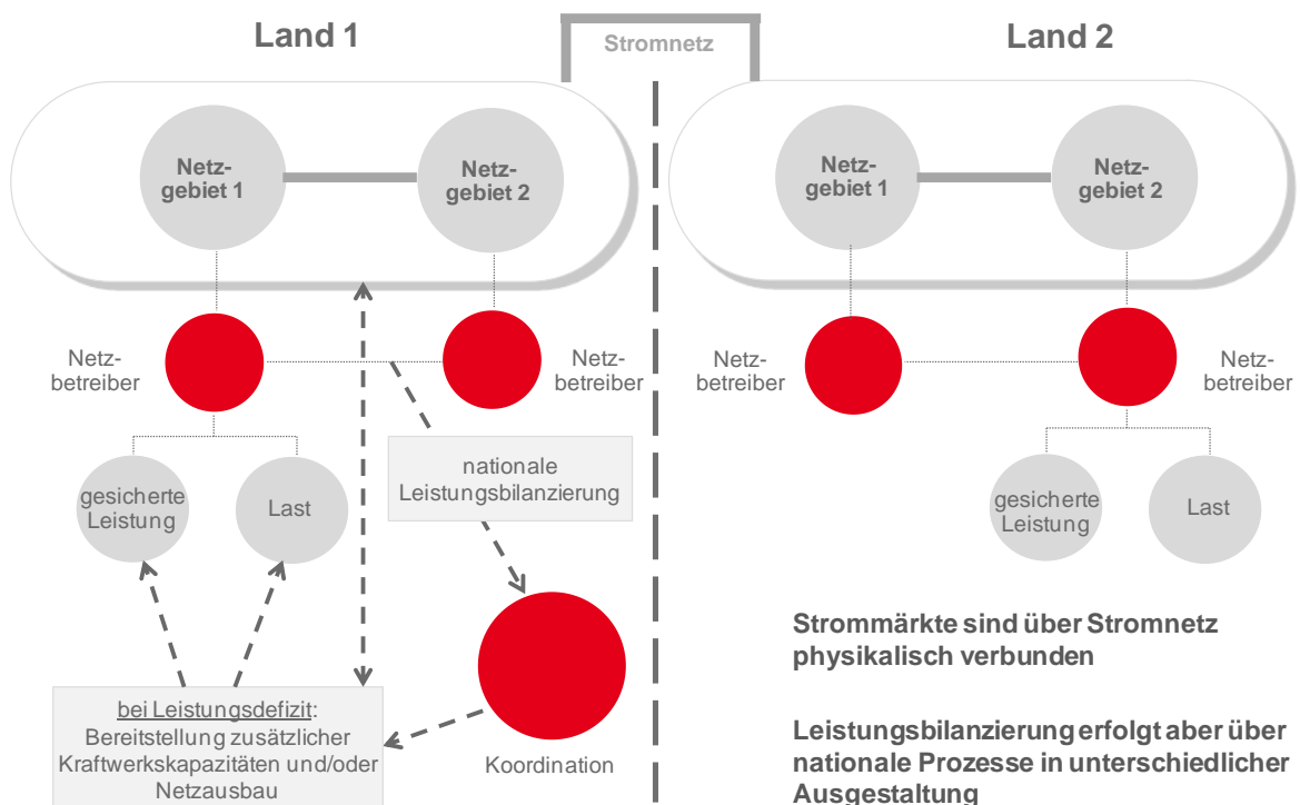
Abbildung 24: Schematische Darstellung des nationalen Leistungsabsicherungsprozesses
