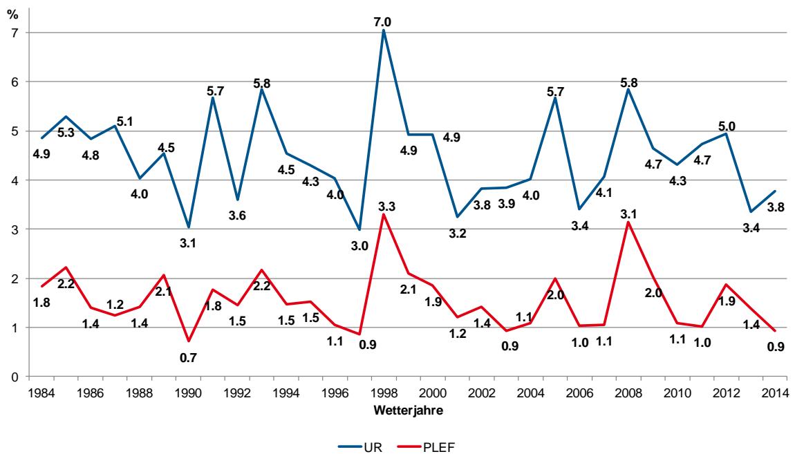
Abbildung 19: Gesicherte (99 %) Windenergieverfügbarkeit in Prozent der installierten Leistung 2030 V3 auf Basis der Wetterjahre 1984-2014
