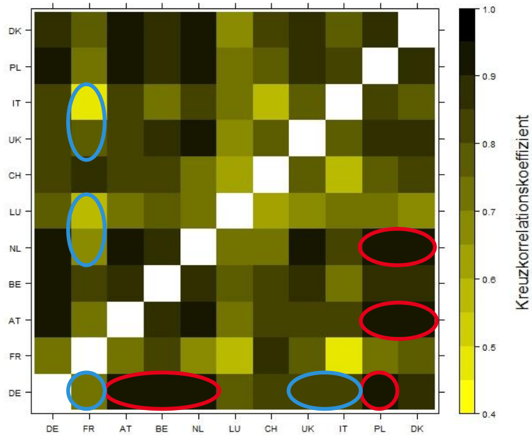
Abbildung 11: Gleichzeitigkeitsanalyse der Last 2011-2013
