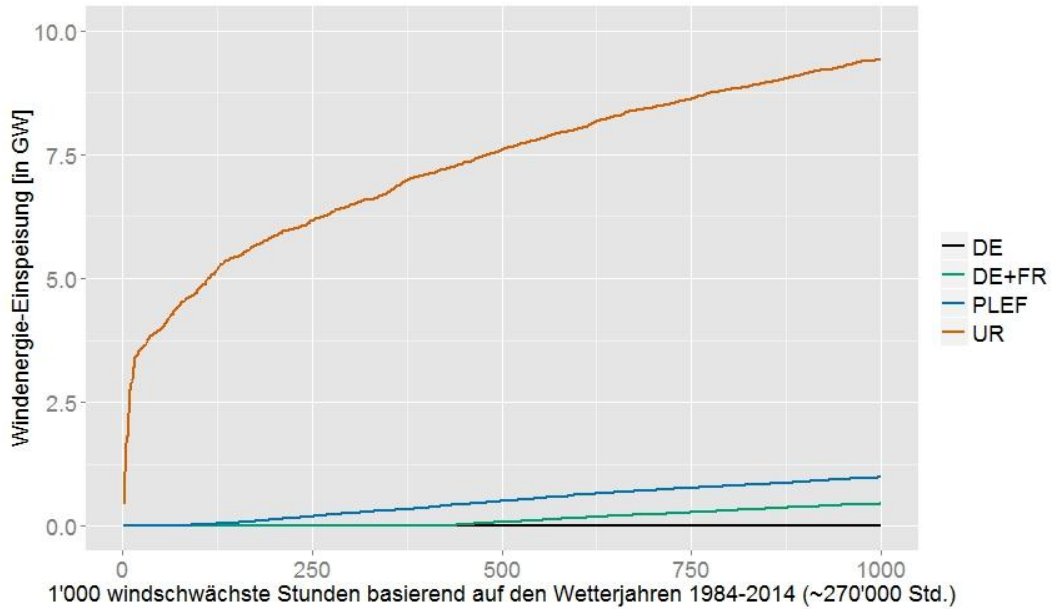
Abbildung 16: Verfügbarkeit der Windenergie in den 1'000 windschwächsten Stunden
