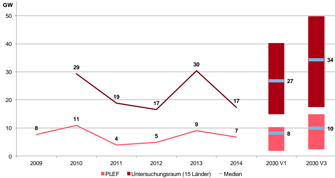
Abbildung 20: Reduktion der residualen Jahreshöchstlast durch gemeinsame Bilanzierung im PLEF und Untersuchungsraum 2009(10)-2014 und 2030
