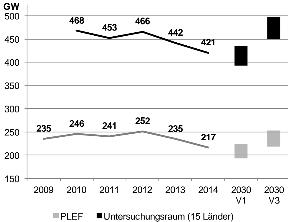
Abbildung 8: Entwicklung der Summe der nationalen Höchstlasten im PLEF und Untersuchungsraum
