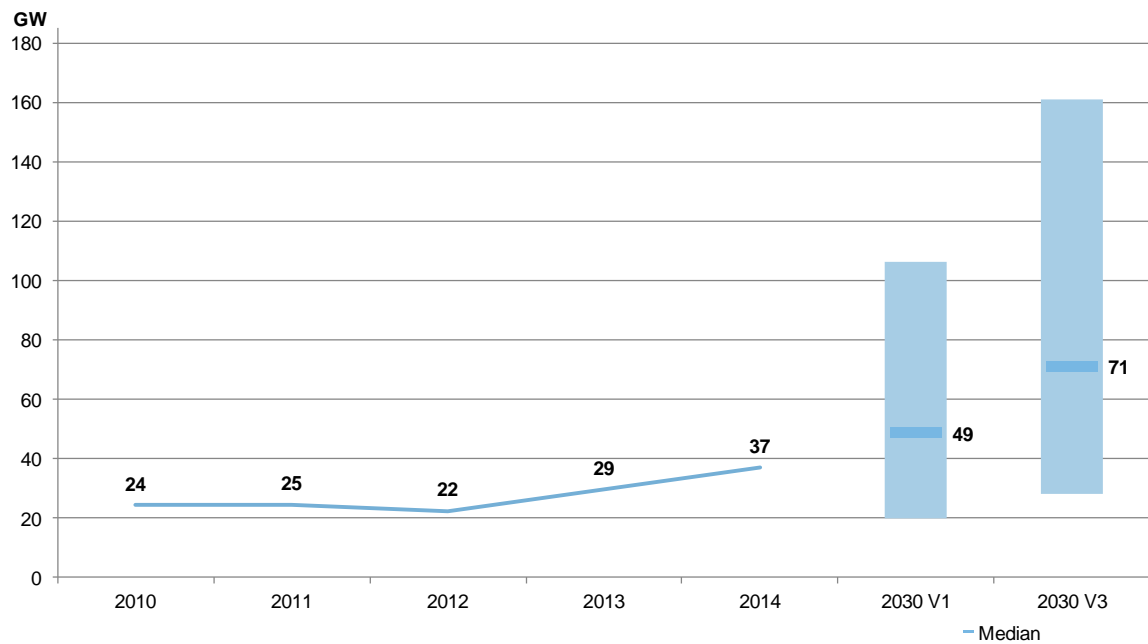
Abbildung 29: Windenergieverfügbarkeit zur Stunde der Verbundhöchstlast im Untersuchungsraum 2010-2014 und 2030
