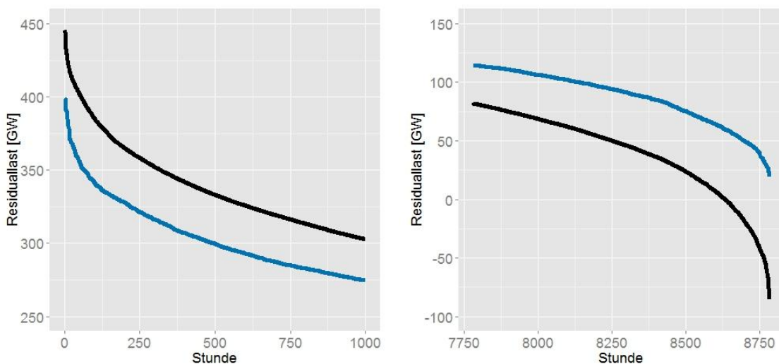
Abbildung 23: Analog zu Abbildung 22 aber für die ersten (links) und letzten (rechts) 1'000 Stunden.
