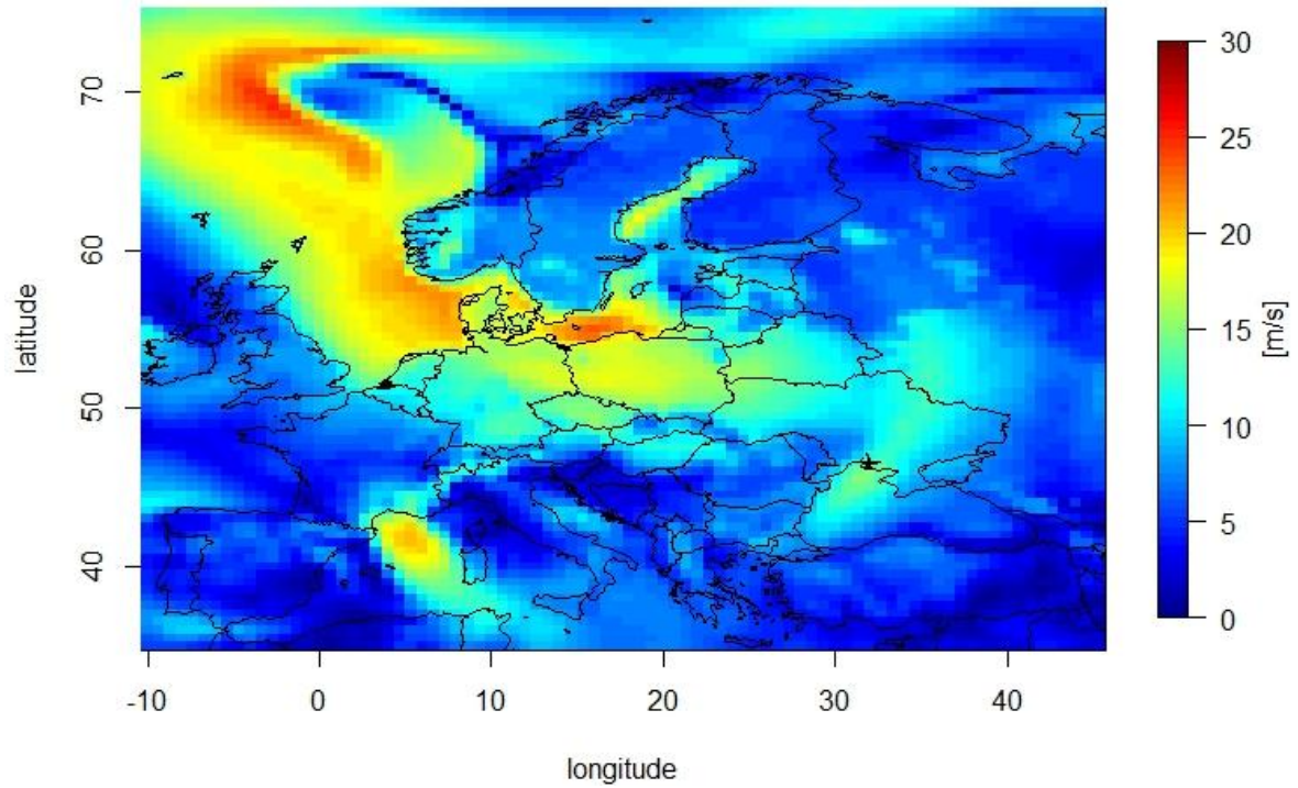
Abbildung 27: Verwendete Reanalyse-Wetterdaten des NASA GES DISC.
