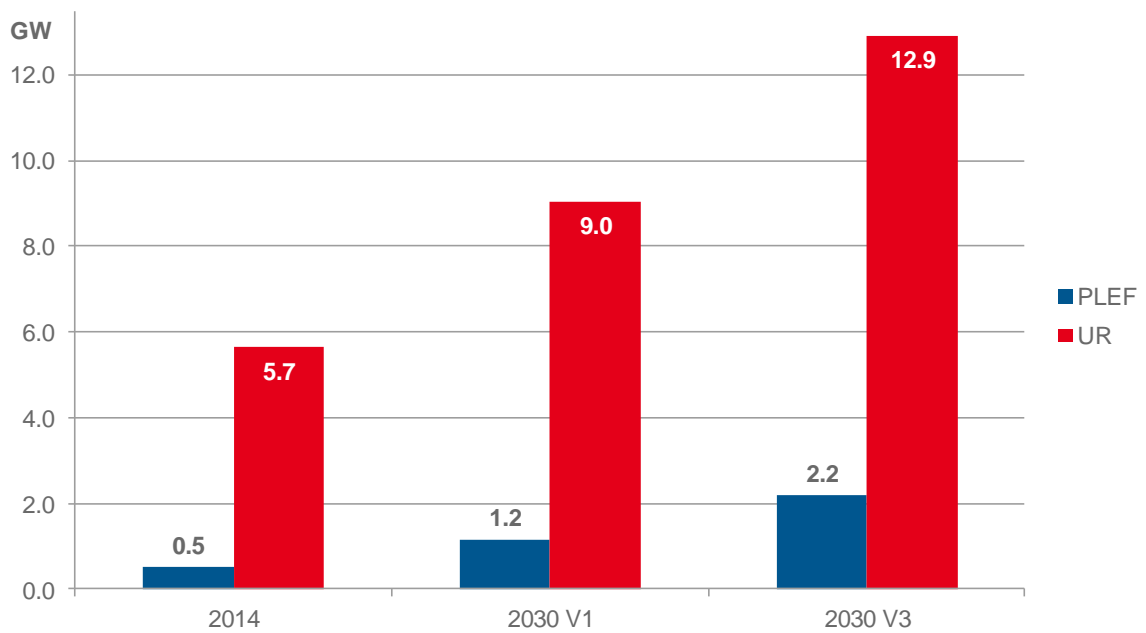
Abbildung 17: Gesicherte (99 %) Windenergieverfügbarkeit in Gigawatt der installierten Leistung 2014 sowie 2030 V1 und V3 auf Basis der Wetterjahre 1984-2014
