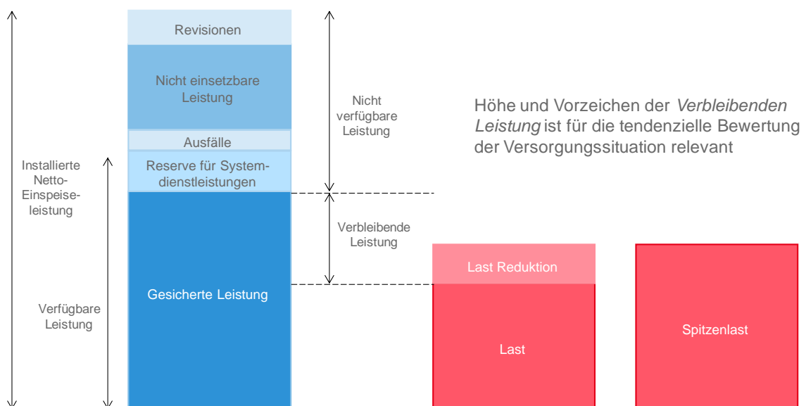
Abbildung 4: Methodik der Leistungsbilanzierung im Ansatz der deutschen Übertragungsnetzbetreiber
