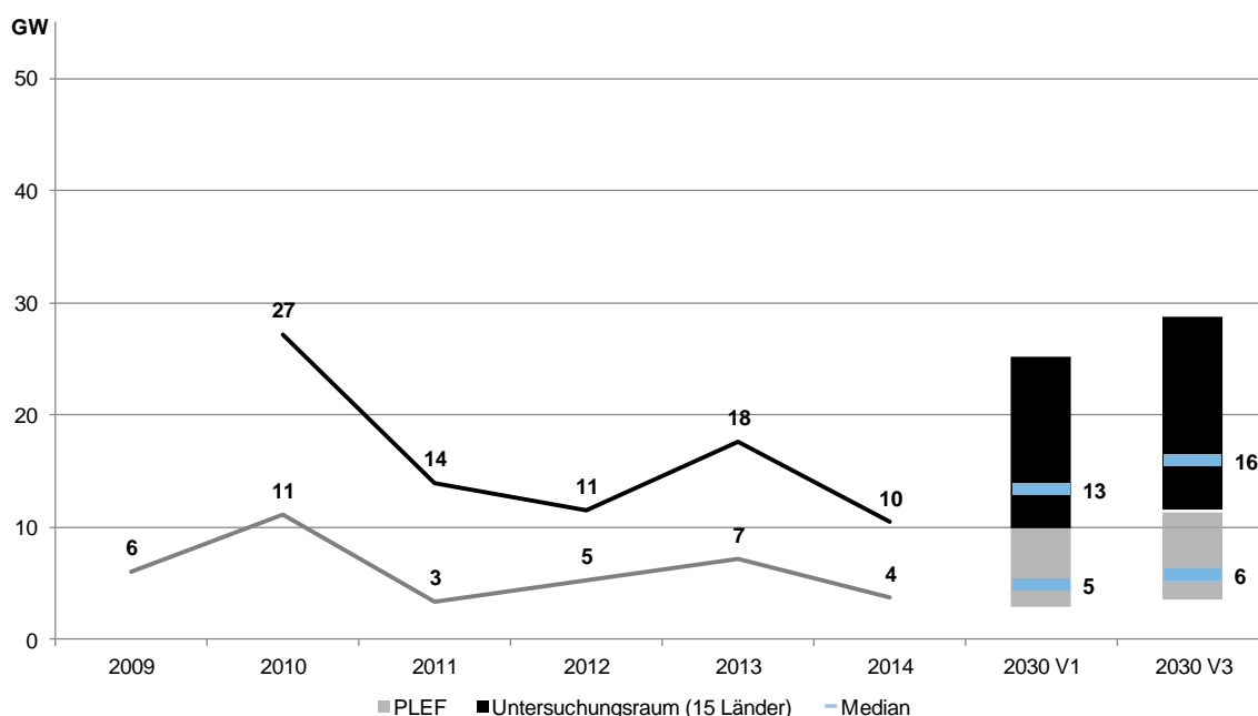
Abbildung 10: Reduktion der Jahreshöchstlast durch gemeinsame Bilanzierung im PLEF und Untersuchungsraum gegenüber nationaler Bilanzierung 2009(10)-2014 und 2030
