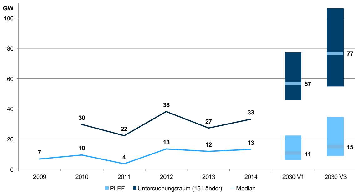
Abbildung 21: Erhöhung der tiefsten residualen Jahreslast durch gemeinsame Bilanzierung im PLEF und Untersuchungsraum gegenüber nationaler Bilanzierung 2009(10)-2014 und 2030
